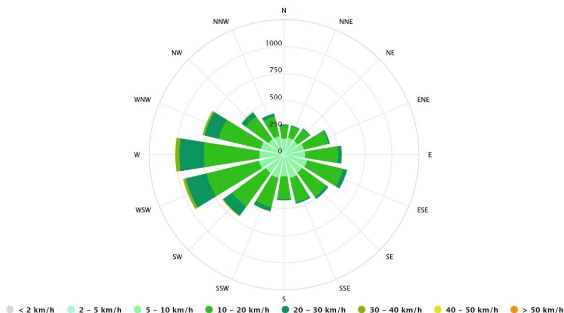
Rysunek 11. Róża wiatrów dla Gminy Międzychód
